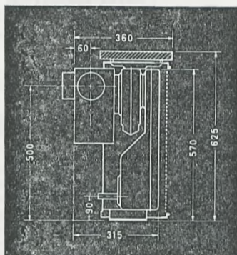
Fig. 1. Skitse af skorstensradiator.
